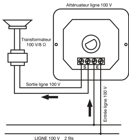
Exemple de connexion en ligne 100 V de 2 fils systèmes
