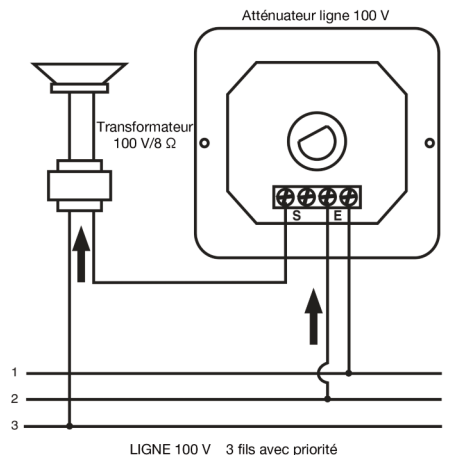
Exemple de connexion en ligne 100 V de 3 fils en de priorité pour appels d'urgence
